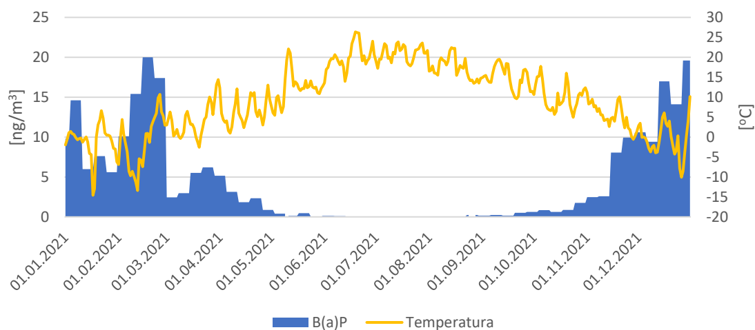
Rysunek 3. Rozkład średniej dobowej stężenia benzo(a)pirenu w pyłe PM10 w roku 2021 w Kaliszu w stosunku do temperatury otoczenia 42
