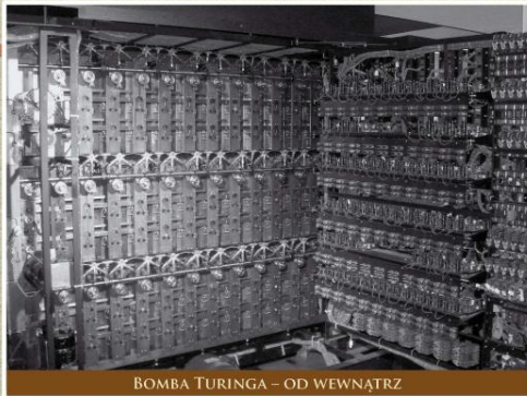
BOMBA TURINGA – OD WEWNĄTRZ
