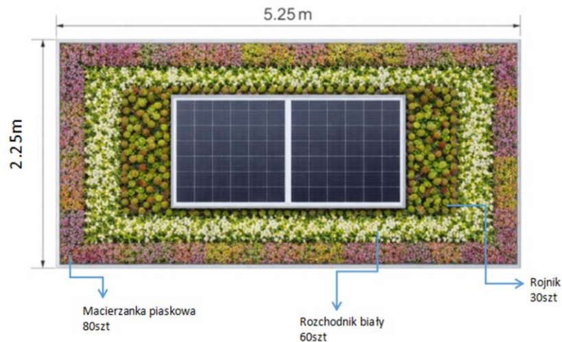
Rzut z góry dachu:
