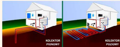
Gruntowa pompa ciepła z kolektorem pionowym i z kolektorem poziomym (www.geobud.pl)
