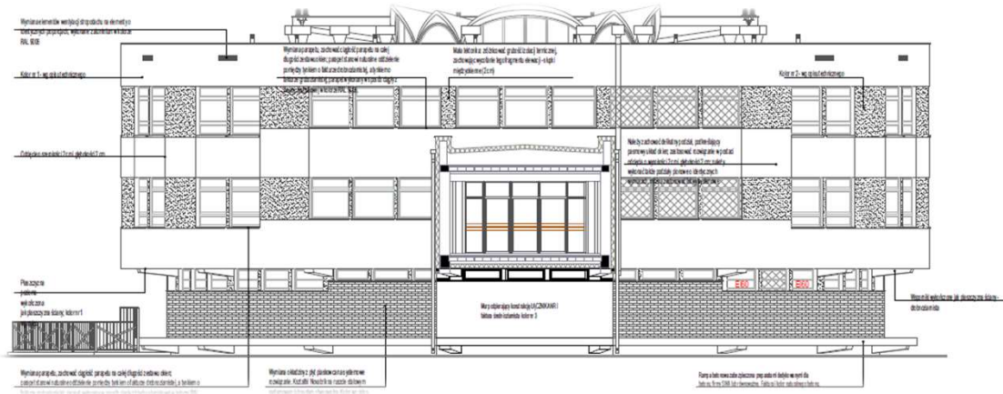
ELEWACJA - ROTUNDA
