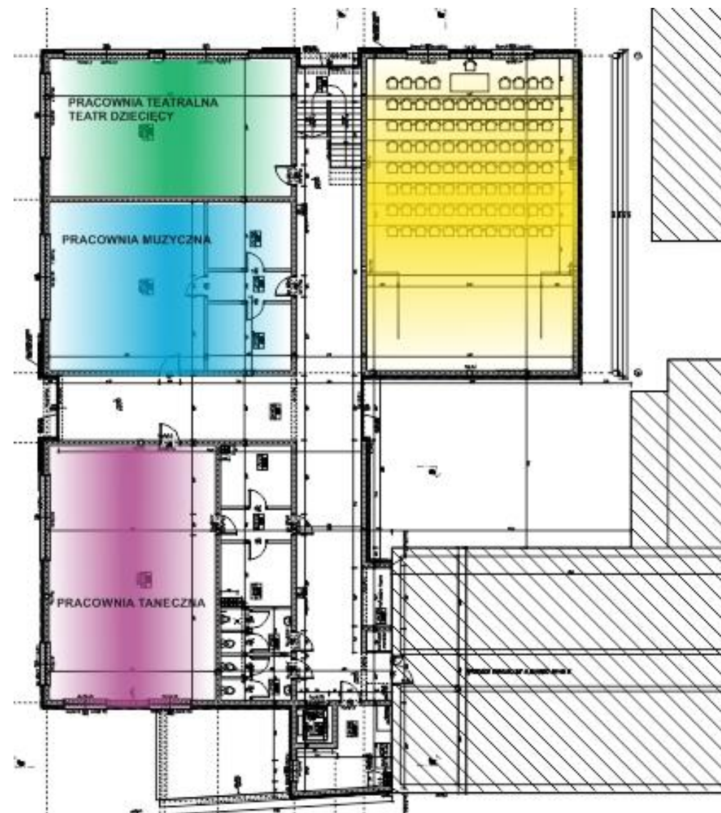
PIĘTRO
